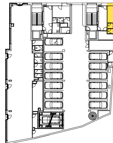
SITUACE OBCHODNÍ JEDNOTKY CELKOVÝ PŮDORYS
